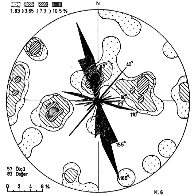
Solmaz ve Haciveliler kavşağı, Granodioritperfir - Grauvak kantağı.
