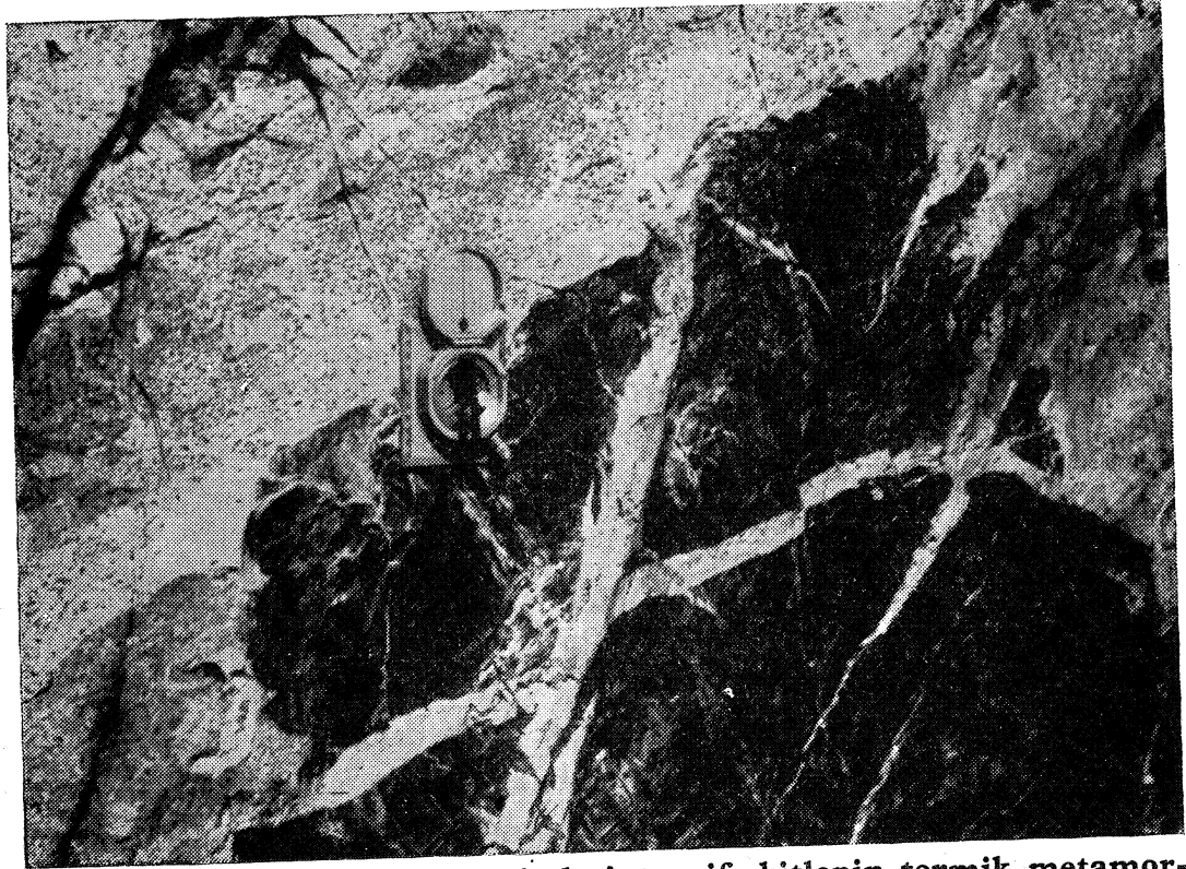
Şek. 6 - Bağıüzü köyü kuzeyinde intruzif kitlenin termik metamorfizmaya uğrattığı yankayaçla olan kontakt durumu.
