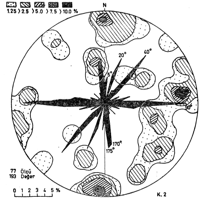
Gazaliburun ile Çaltı köprüsü arası Granodiorit.
