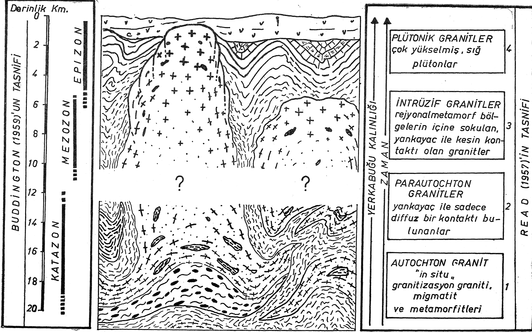
Şek. 9 - Granitizasyonu ve intruzyon kabiliyeti kazanmış bir kitlenin yerkabuğunun çeşitli derinliklerdeki durumunu gösterir şema. [Read (1957) ve Buddington'dan (1959) istifade ederek çizilmiştir].
