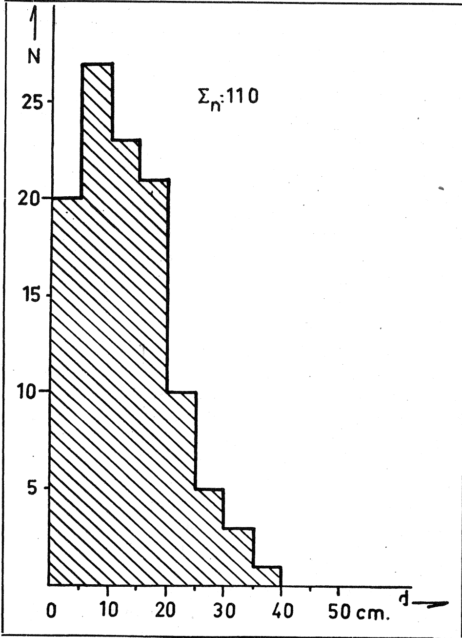
Şek. 4 - Kozak aplitleri, damar kalınlıkları grafiği. (Toplam aplit sayısı E_n 110.)
