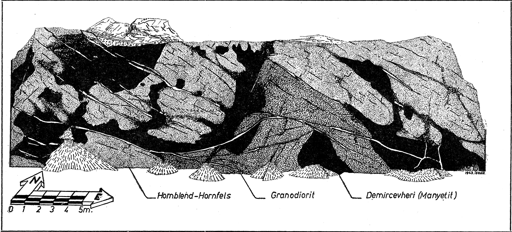
Şek. 8 - Karahayit köyü güneyinde granodiyorit kontaktındaki hornfels teşekkülü ve cevherleşme.
