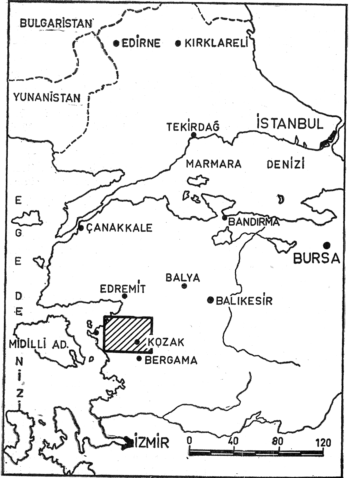
Şek. 1 - Etüd bölgesini gösteren indeks haritası.
