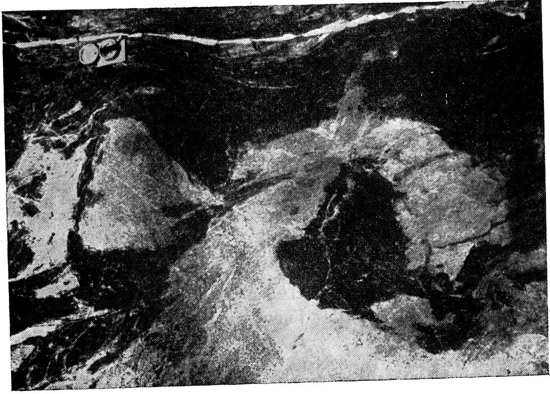
Şek. 5 - Bağıüzü köyü kuzeyinde agmatik yapı gösteren kontakt zonu.
